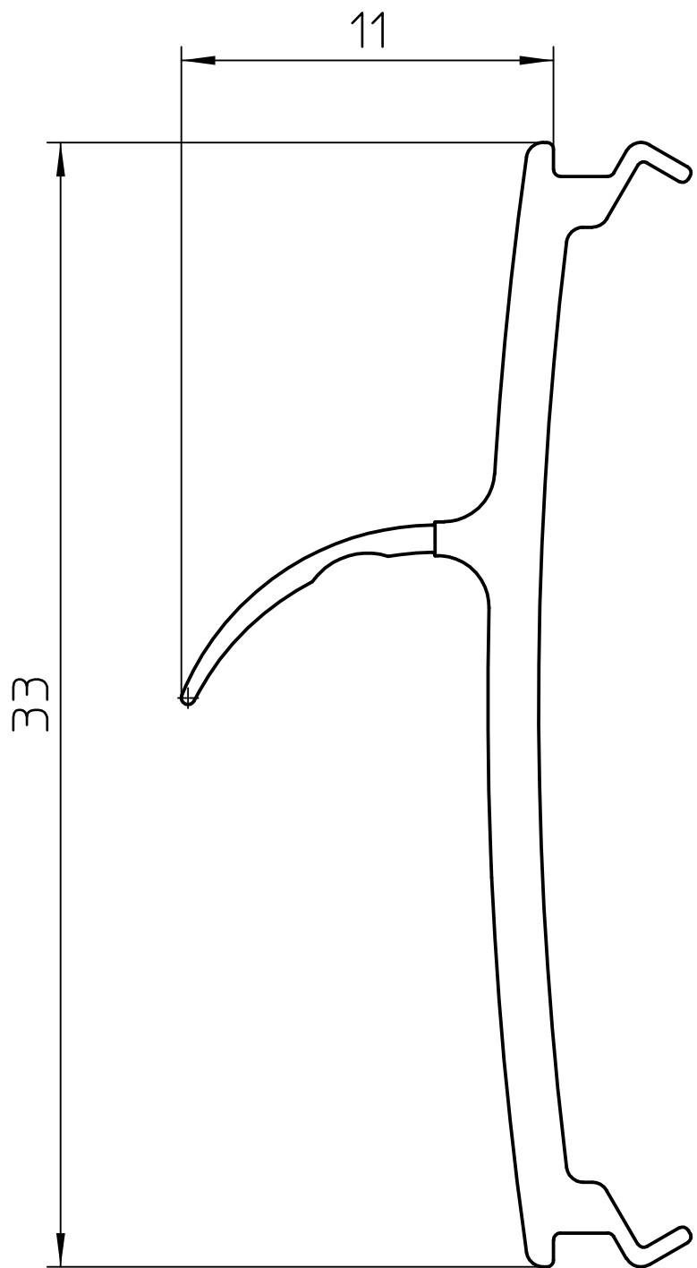
Seitenansicht Side View M 5:1
