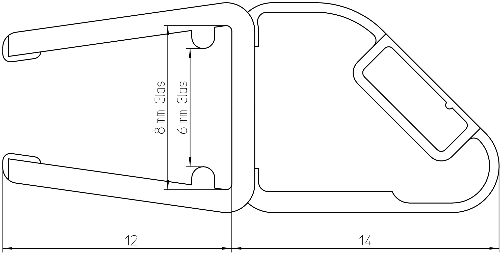
Seitenansicht Side View M 10:1
