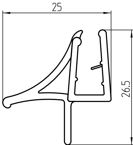
Seitenansicht Side view M2:1
