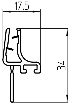
Seitenansicht Side view M1:1
