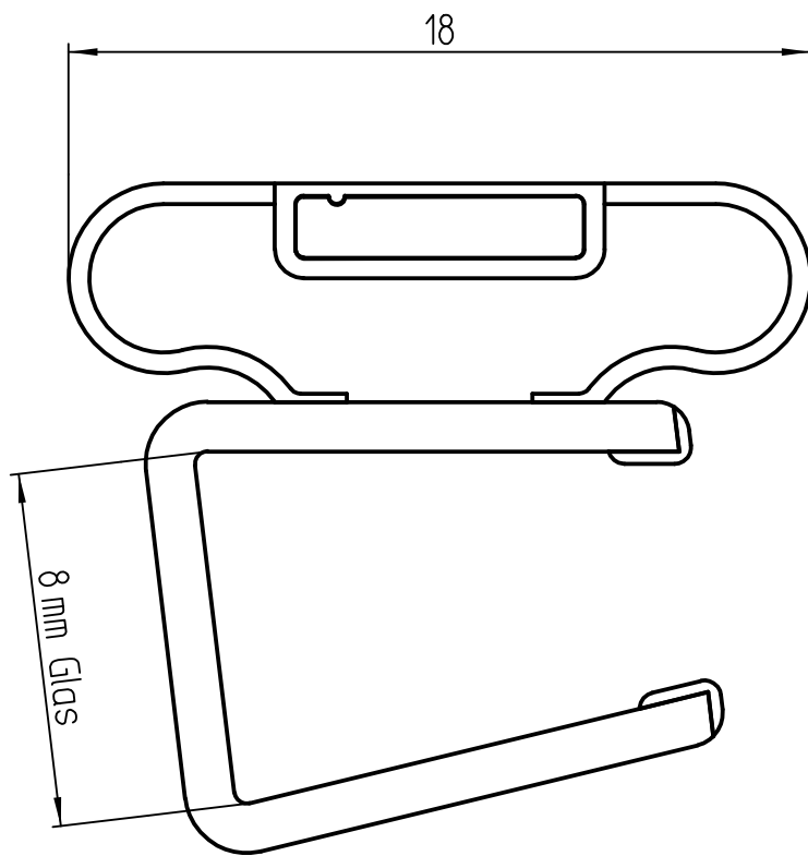
Seitenansicht Side View M 5:1
