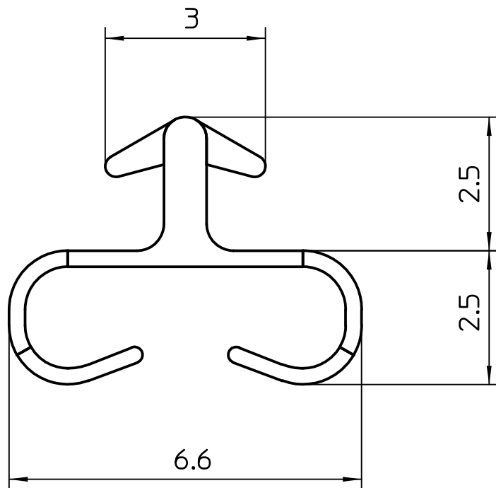
Seitenansicht Side View M 10:1
