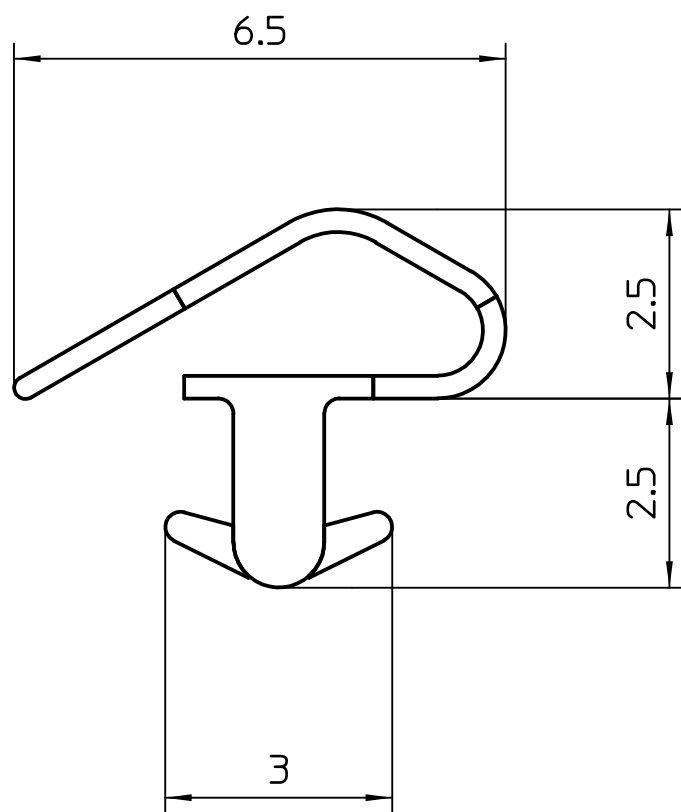
Seitenansicht Side View M 10:1
