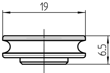
Seitenansicht Side view M2:1
