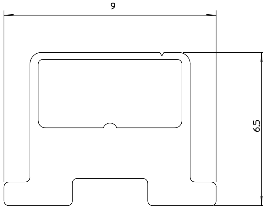
Seitenansicht Side View M 10:1
