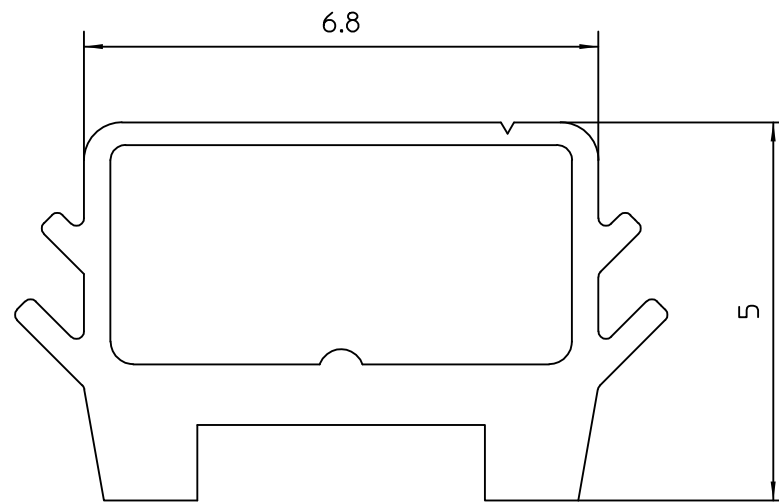
Seitenansicht Side View M 10:1
