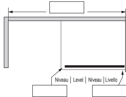
Nischenbreite für Traverse Typ B ( 180° ) Width of recess for stabilising bar typ B ( 180° ) Largeur de la niche pour traverse typ B ( 180° ) Larghezza de la nicchia per traversa typ B ( 180° )
