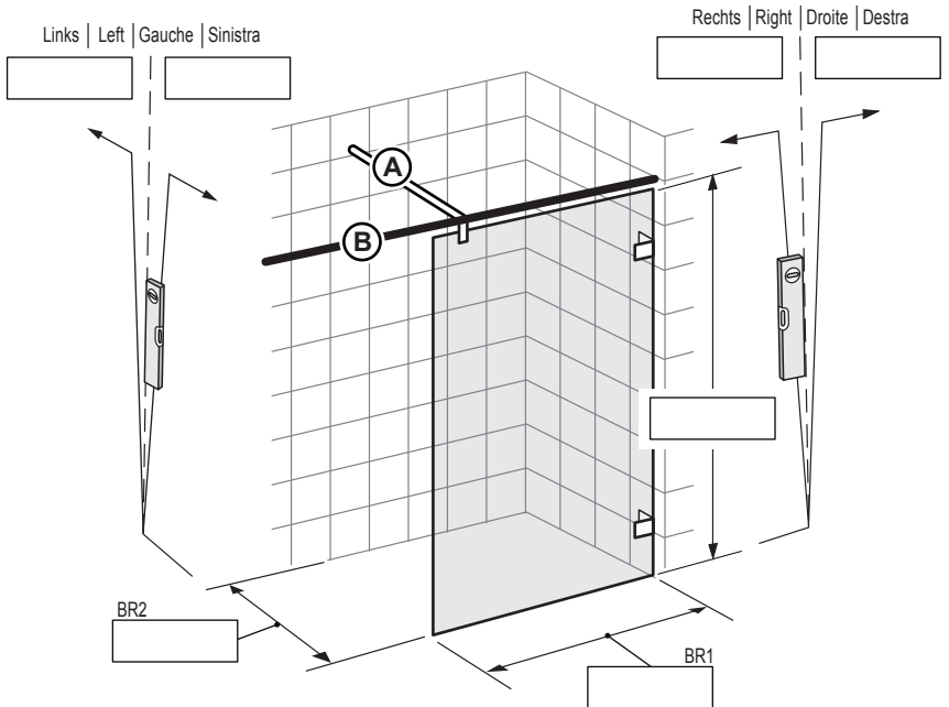
Nischenbreite für Traverse Typ B ( 180° ) Width of recess for stabilising bar typ B ( 180° ) Largeur de la niche pour traverse typ B ( 180° ) Larghezza de la nicchia per traversa typ B ( 180° )
