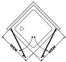
Bovenaanzicht
