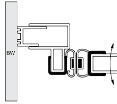
Sokkelprofiel voor montage tegen bad
